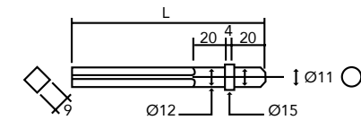
11 MM FCH-20-1F ○
